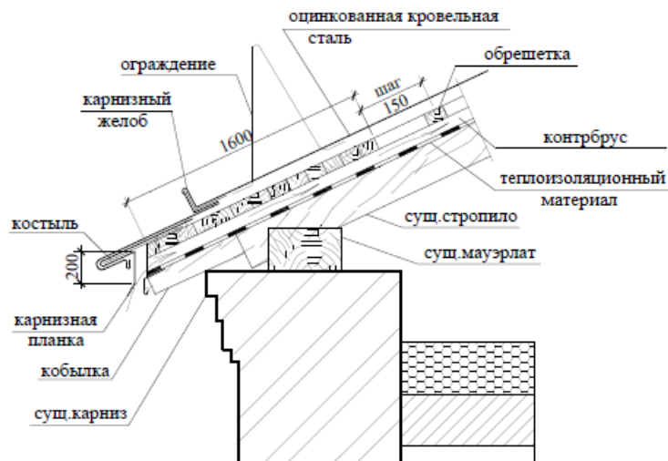
Рис 10-2. Узел устройства карнизного свеса. Вариант 2.
