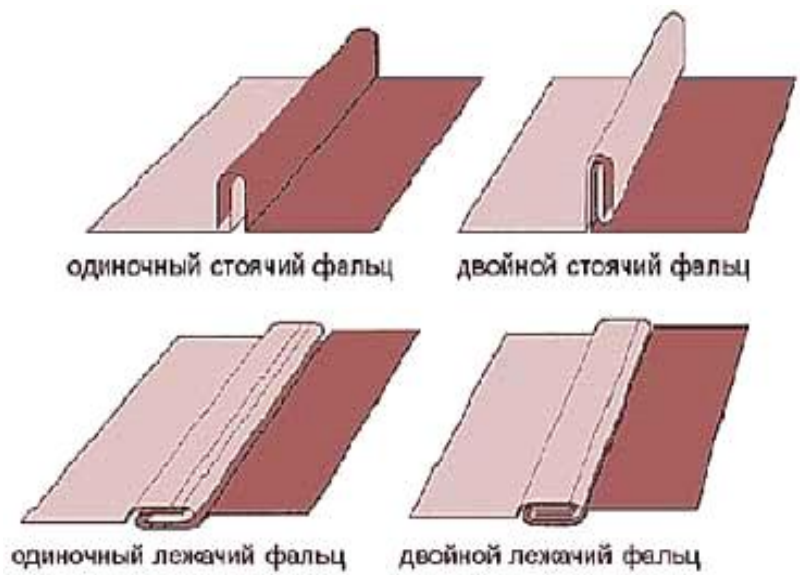
Рис.1. Одинокый и двойной фальц
