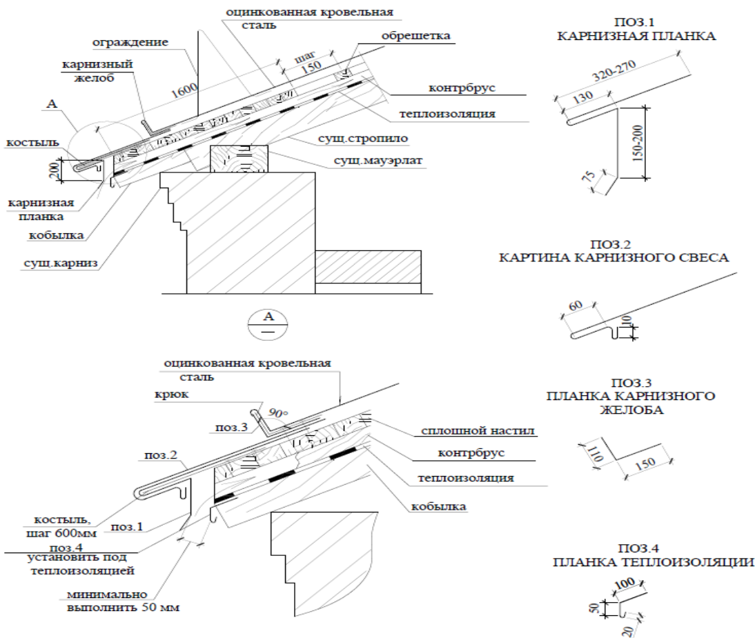
Рис.6. Узел устройства карнизного свеса. Спецификация узлов.
