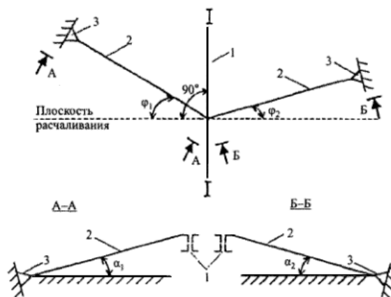
1 - ферма; 2 - расчалка; 3 - якорь
